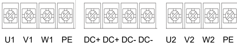
图 2-1 DS20270HA 主回路端子
