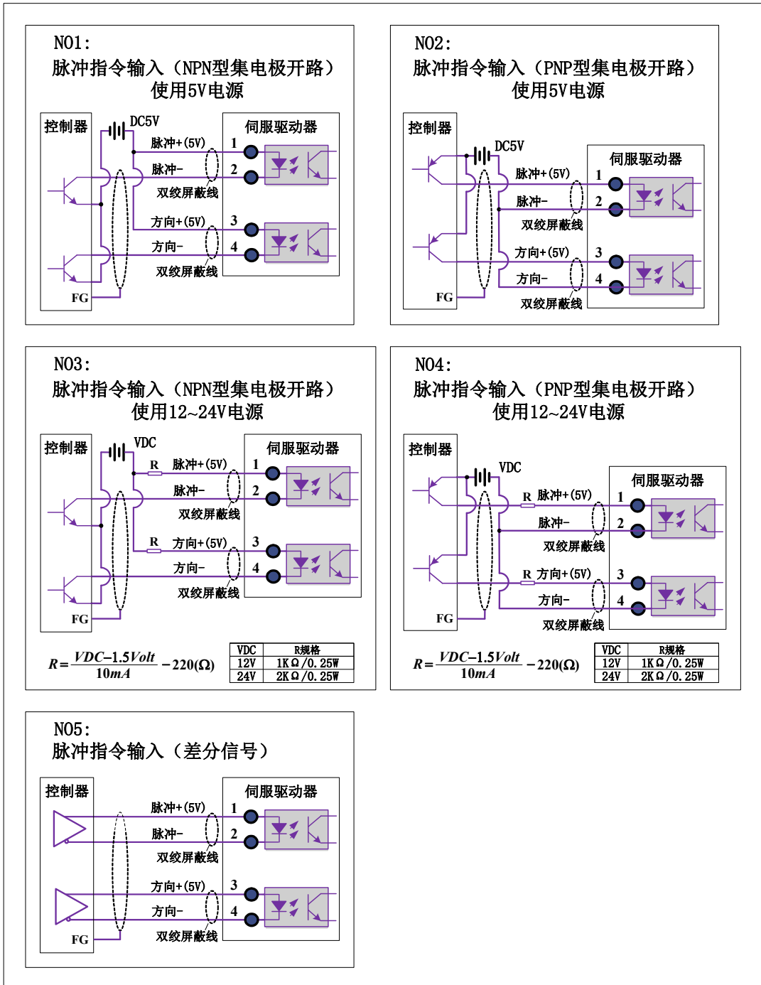
图 2-7 脉冲指令输入接线图
