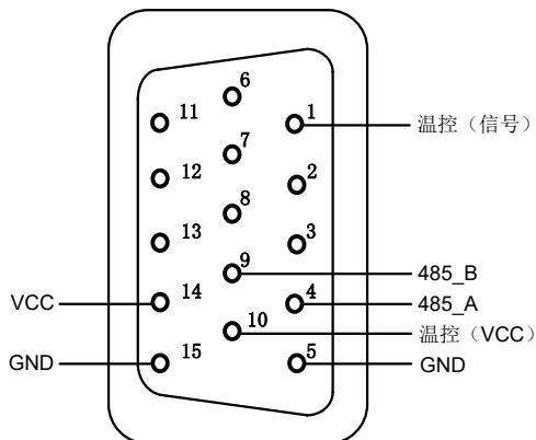
DS20270HA 编码器接口的管脚定义
